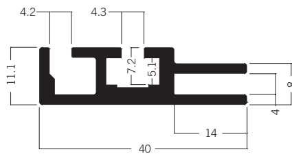
M 1930 Spannrahmenprofil für Leuchtrahmen 40 mm 3.41 kg | 6000 mm
