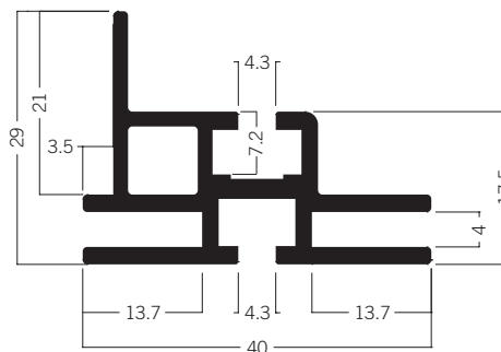
M 1970 Spannrahmenprofil für Leuchtrahmen 40 mm 4.34 kg | 6000 mm
